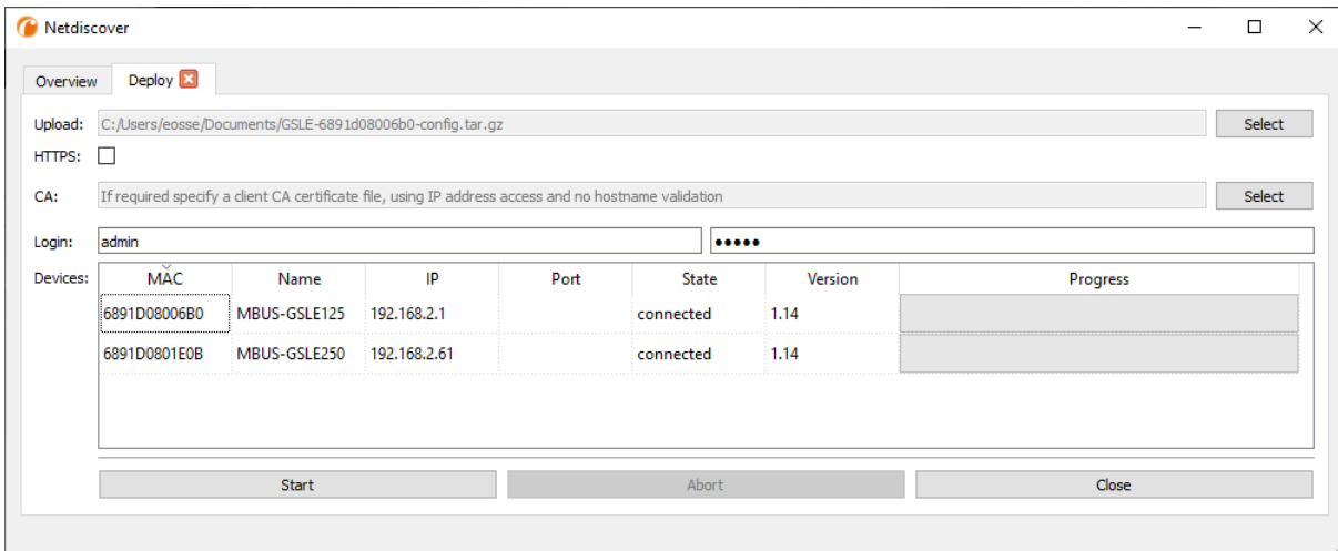
Figure 11 – Déploiement en bloc sous l'outil Netdiscover
