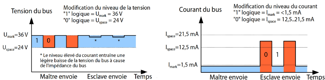
Figure 26 – Signalisation sur le M-Bus
