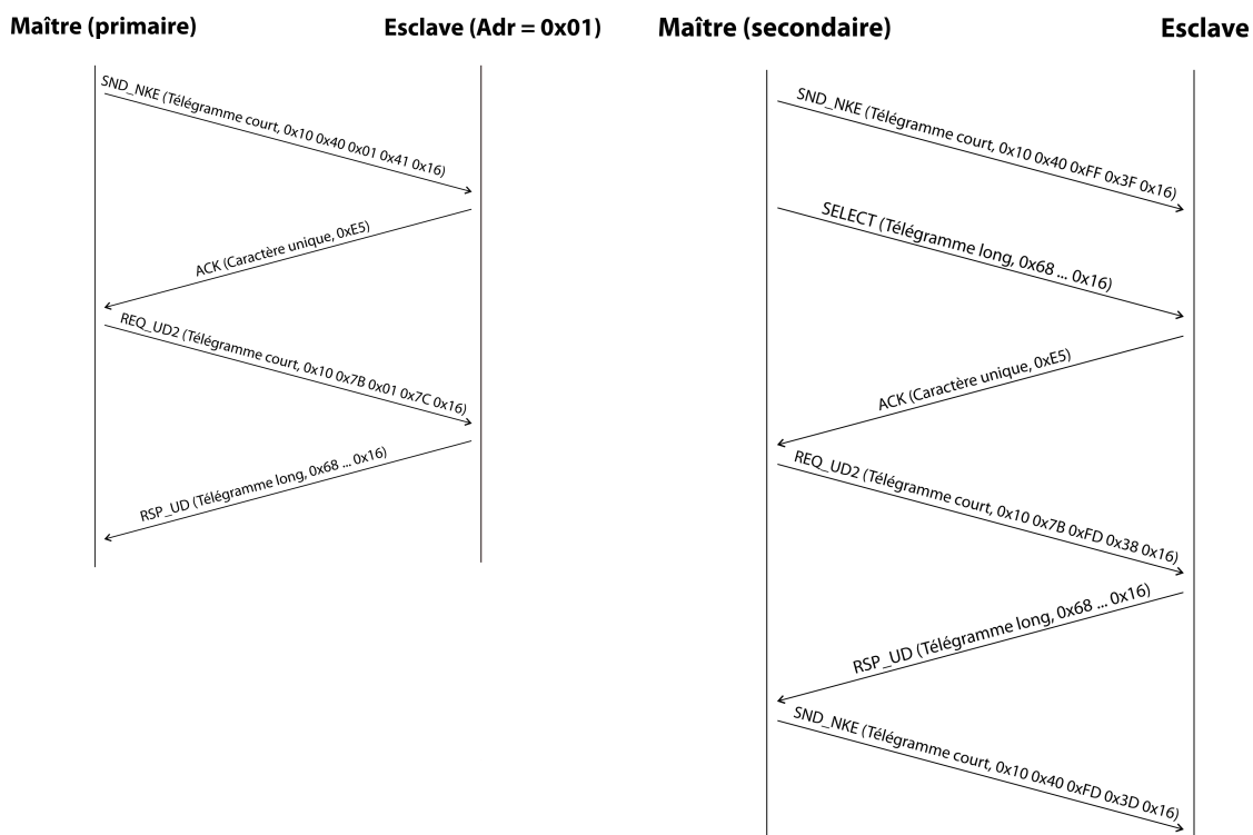
Figure 27 – Exemple de l'adressage primaire et secondaire en comparaison
