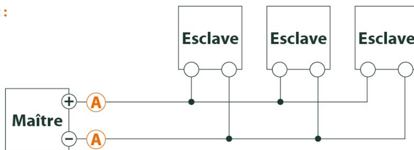
Figure 28 – Dépannage chez le M-Bus à travers des mesures avec multimètre
